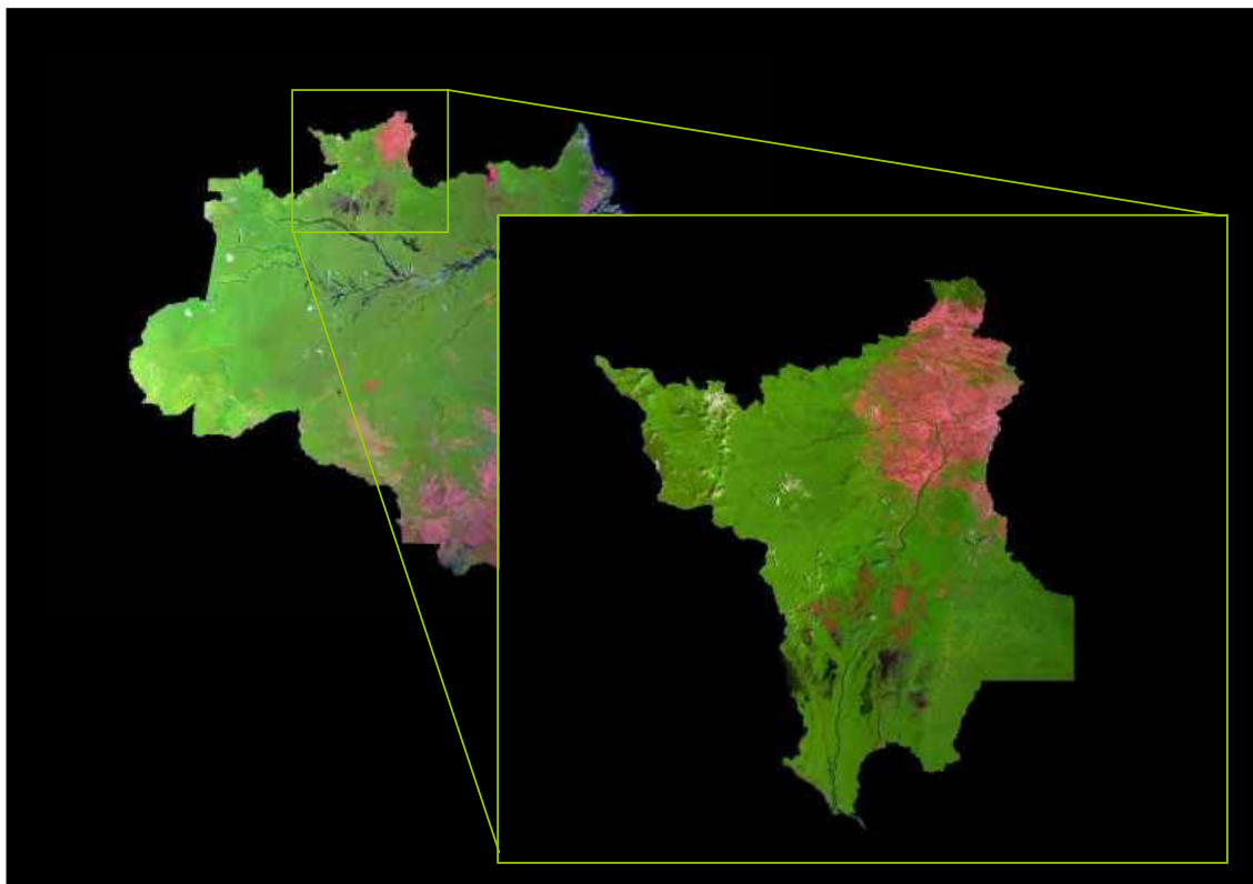
Figura 1 – Roraima no contexto da Amazônia brasileira - as savanas são representadas pela coloração rosa no setor norte-nordeste do Estado (Fonte: http://www.cnpm.embrapa.br-Coleção Brasil Visto do Espaço )
